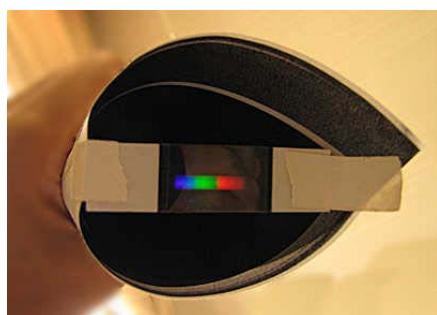
室外光のスペクトル
